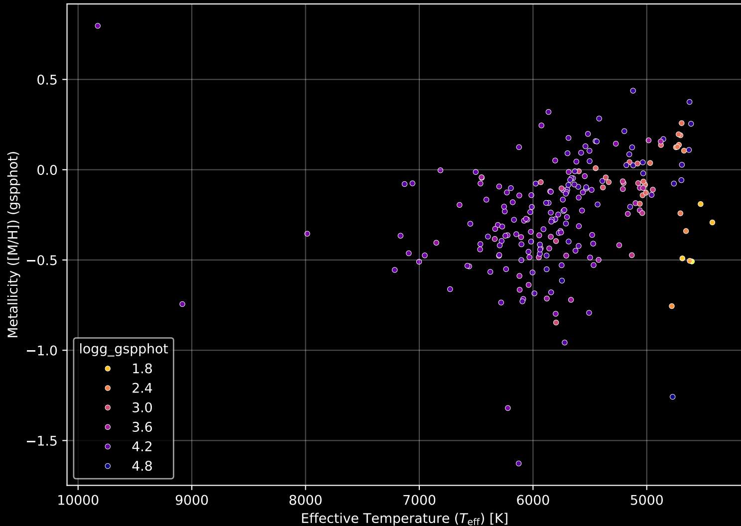
GALAH DR4 Field: [7151] Stellar Population Parameters (n= 220)
