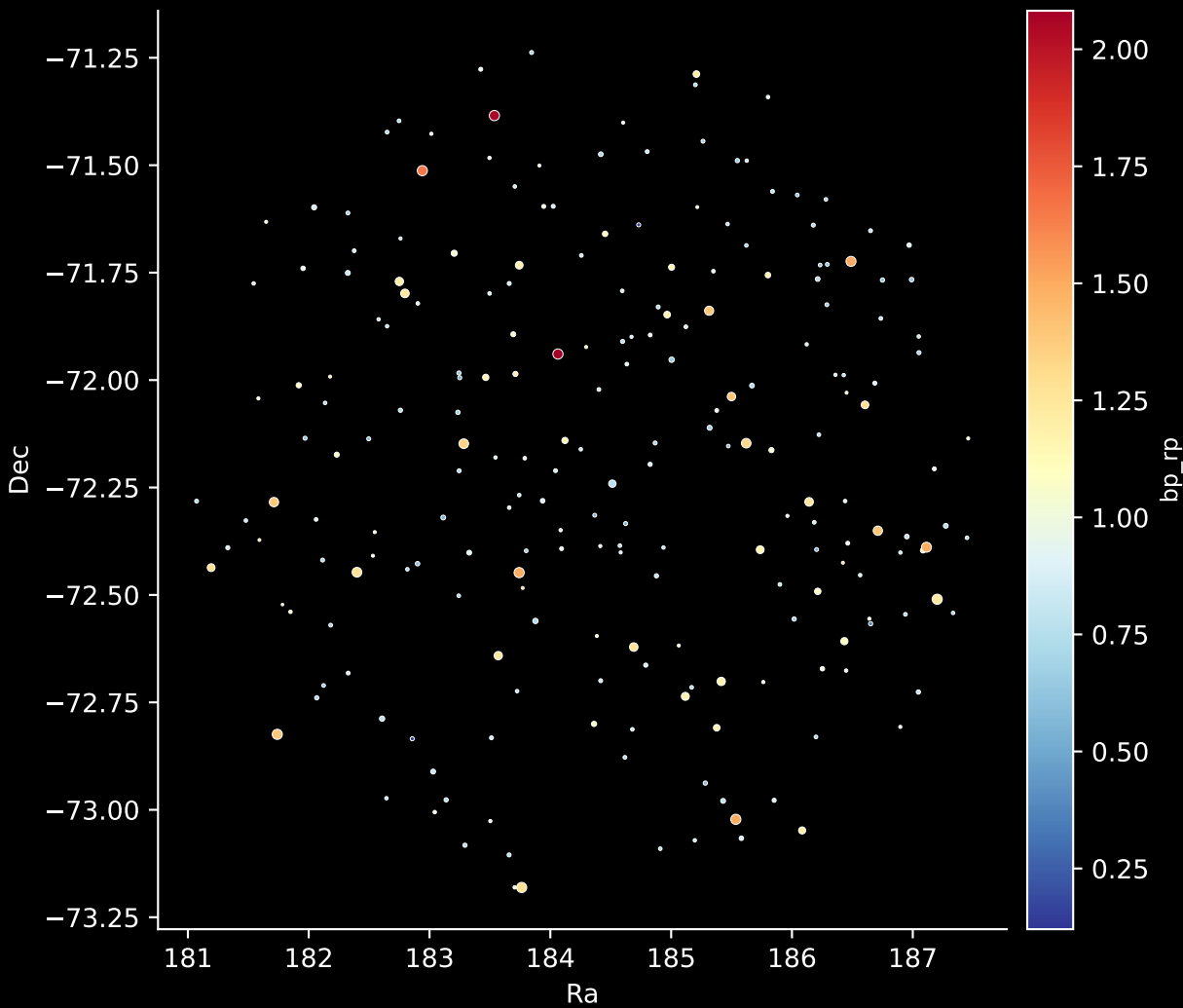
GALAH DR4 Field: [7151] Stars: 220
